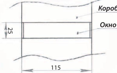
ОКНО ДЛЯ ПОДАЧИ НЕОЧИЩЕННЫХ ЯГОД (ВИД Б)
