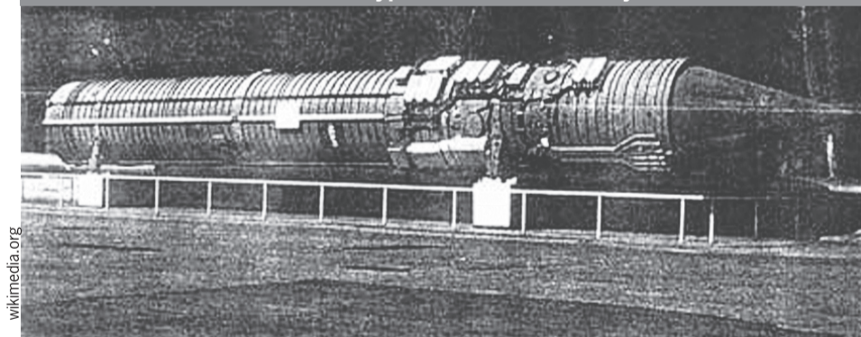
Так выглядела командная ракета 15А11 системы «Периметр», когда ее выпускали в днепропетровском КБ «Южное». 6 из 7 испытаний на Байконуре в 80-е годы были успешными.
