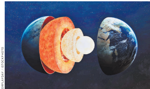
Профессор Артем Оганов: У молодой Земли не было ни ядра, ни мантии, а ее химический состав был однородным...
