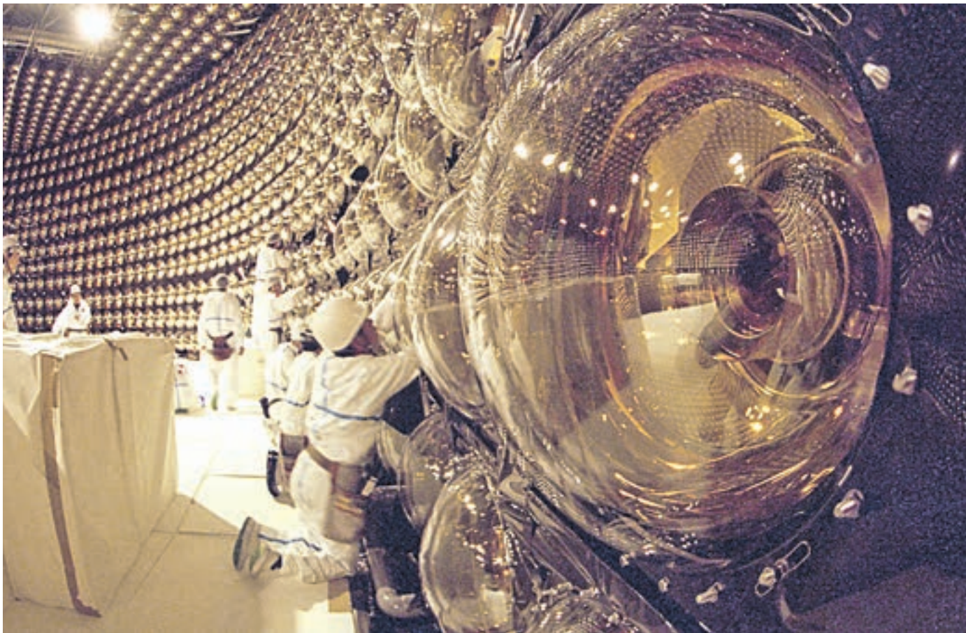
15 марта 2013 года. Так ловят нейтрино. Японская нейтринная обсерватория Super-Kamiokande находится под землей на глубине километра. Стены цилиндра диаметром 39 метров и высотой 41 метр покрыты 11 146 вакуумными уловителями. Каждый стоит более 3000 долларов. Размах впечатляет
